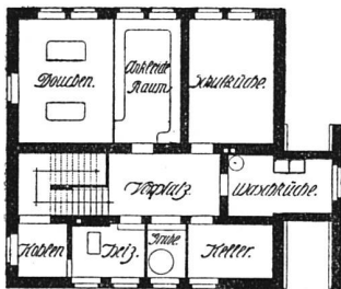
Das Sekundarschulhaus in Oberuzwil (Kanton St. Gallen). — Architekt (B. S. U.) Paul Truniger in Wil Grundrisse des Kellers, des Erdgeschosses, des Obergeschosses und des Dachstokes. — Maßstab 1:400
