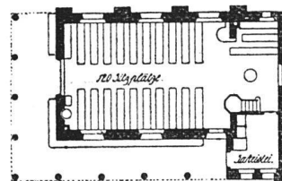
Grundriß 1:400
