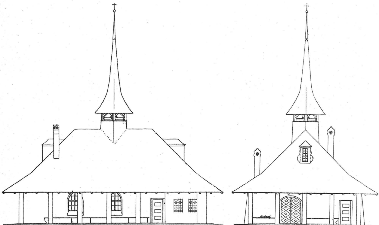
Seitenfassade Maßstab 1:200 Eingangsfassade Die Kapelle auf der Grimmialp. — Architekten B. S. A. Joss & Klausner in Bern
