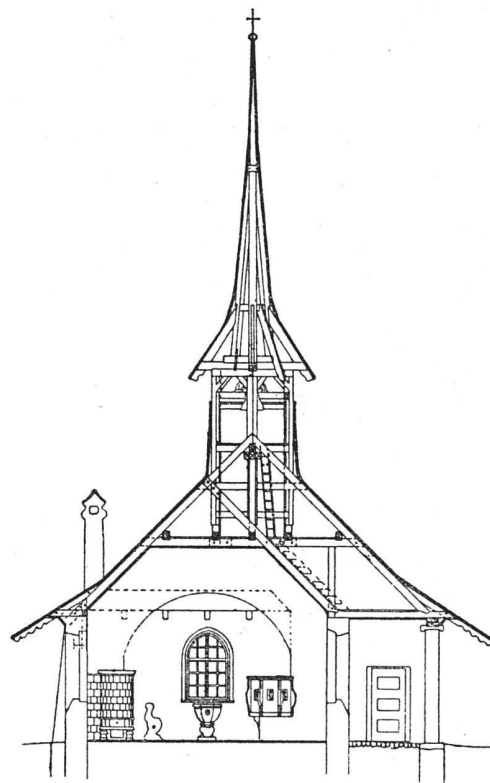
Querschnitt 1:200
