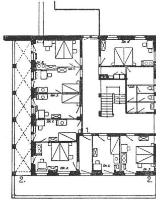
Obergeschoss-Grundriß
