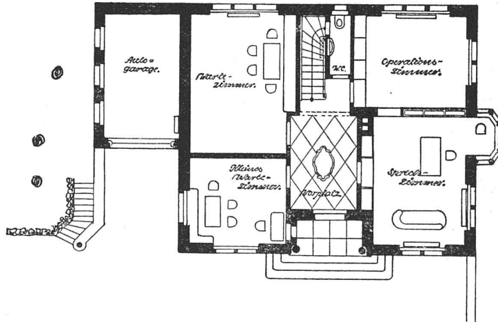
Erdgeschoss-Grundriß Maßstab 1:200
