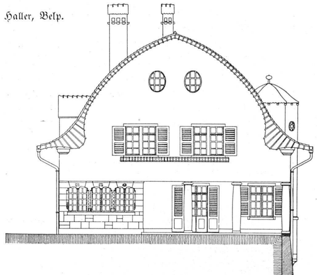
Südfassade.
