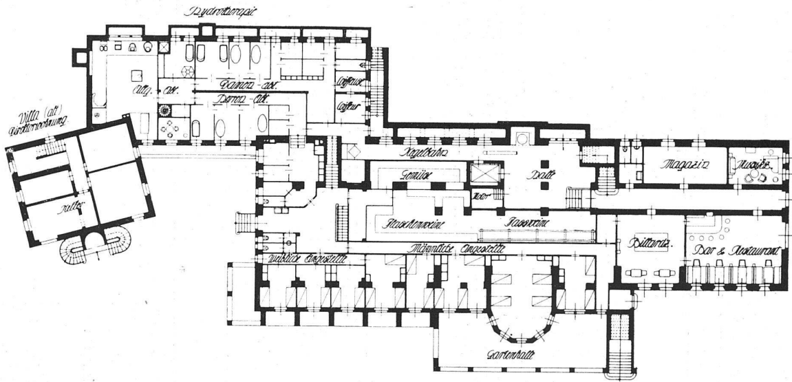
Grundriß Kellergehoß
