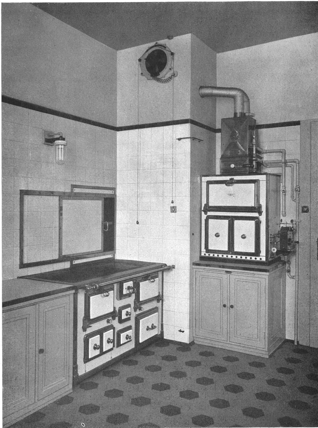
Aus der Küche der Villa Wegelin-Hauser in St. Gallen. Senking Kohlenherd, darüber Wärmeschrank, daneben Heisswasserapparat und kombinierte Spieß- und Grill-Einrichtung mit Backofen.
