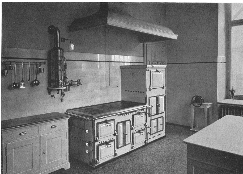
Aus der Küche der Villa Windegg in Zürich. Senking-Gasherd mit angebautem Spiess- und Grill-Apparat.
