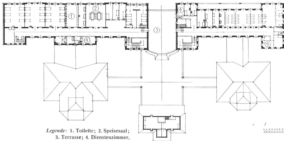
Frauenklinik und Kinderspital in Lausanne. — Grundriss des ersten Stockwerkes.
