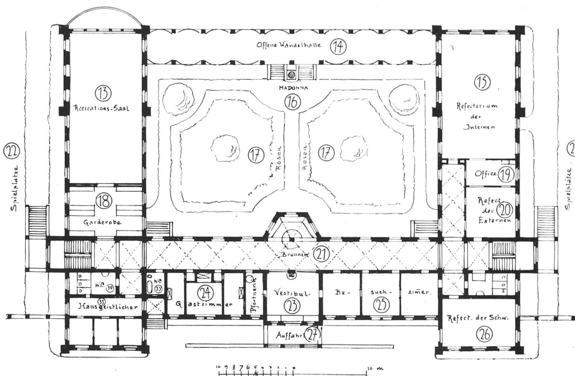
Institut «Stella maris» in Rorschach. — Parterre-Grundriss. Architekt A. Hardegger, St. Gallen.
