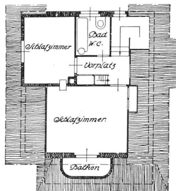
1. Stock-Grundriss.
