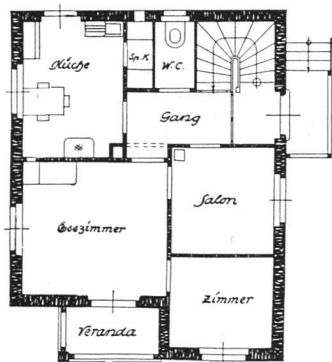
Parterre-Grundriss.
