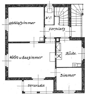
Erstes Geschoss - Grundriss.
