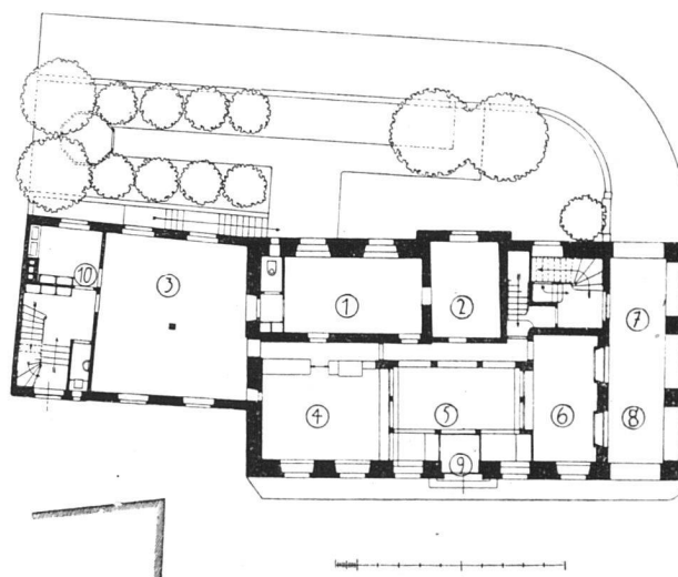
Bankhaus Wegelin & Co., zum Nothveststein, St. Gallen. Grundriss des Erdgeschosses. — Architekten: von Ziegler & Balmer, St. Gallen.
