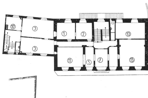
Bankhaus Wegelin & Co., zum Nothveststein, St. Gallen. Grundriss des ersten Stockes. — Architekten: von Ziegler & Balmer, St. Gallen.
