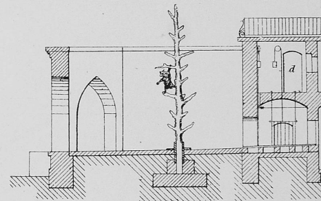
Schnitt A.B.
