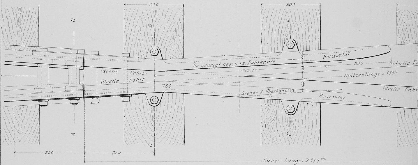
Grundriss
