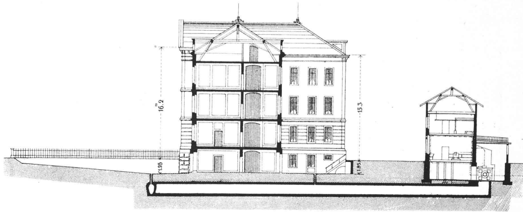
Längenschnitt 1:500.
