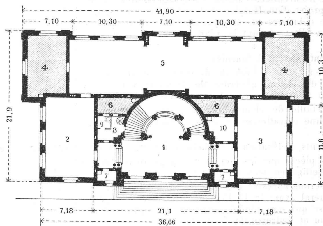
Grundriss.
