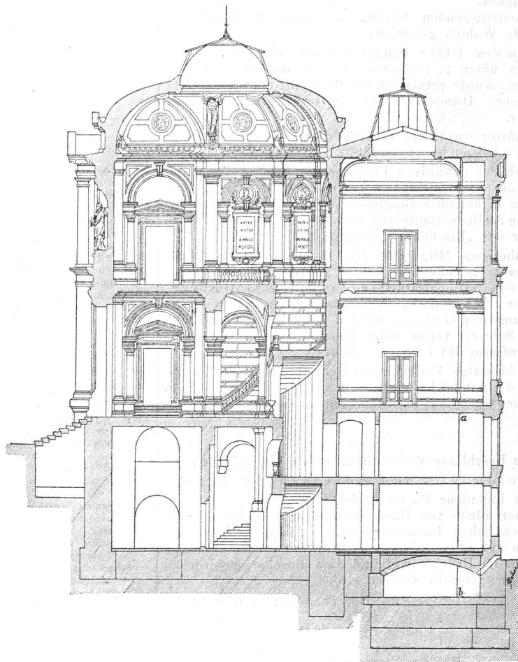
Querschnitt.
