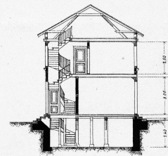
Querschnitt A-B
