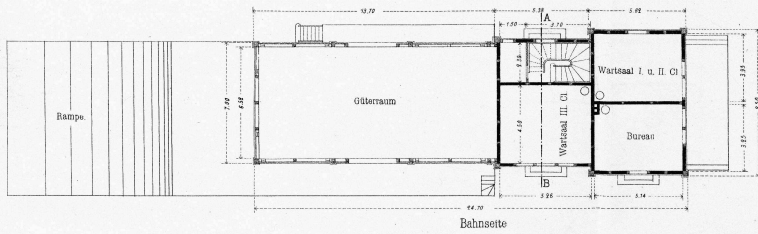
Grundriss des Erdgeschosses
