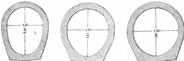
Jetziges Wolfbachprofil.
