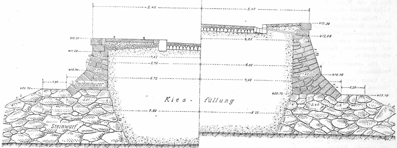
Fig. 3. — Normalprofil des mittleren Dammes.
