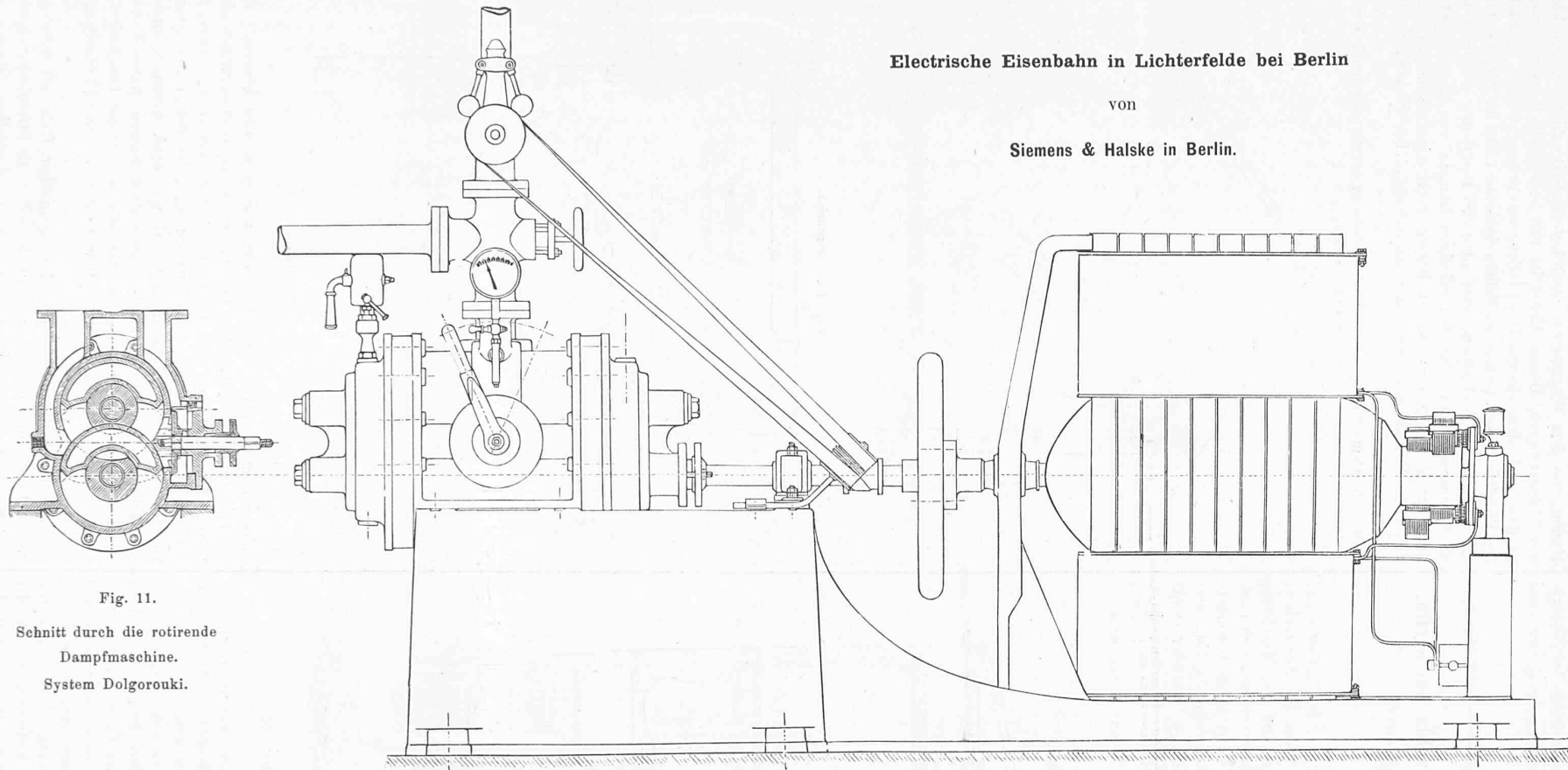
Fig. 12. Betriebsmaschine für die electrische Eisenbahn.
