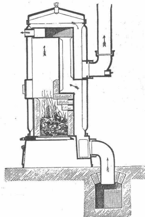
sowie nach eigenem System, zum Heizen von Räumen bis 5000 m³ Inhalt.
