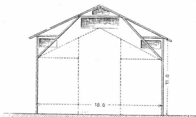
Hauptbau, Eckpavillon (Schnitt.)
