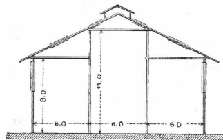
Hauptbau, grosse Verbindungshalle (Schnitt)
