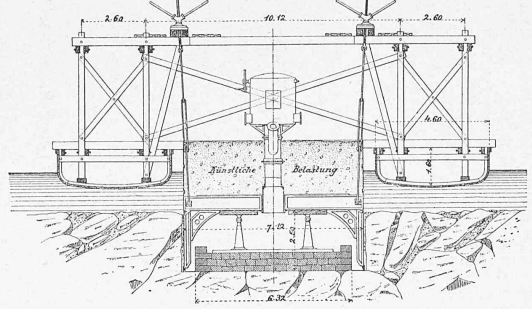
Fundation des 2 ten Pfeilers
