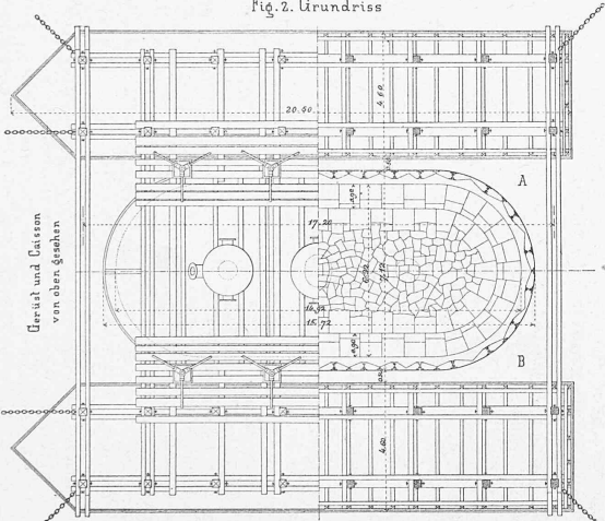
a Luftschleuse für die Einführung der Quader. A Horizontalschnitt unterhalb der Decke des Caissons. B Horizontalschnitt nach Beendigung der Mauerung.
