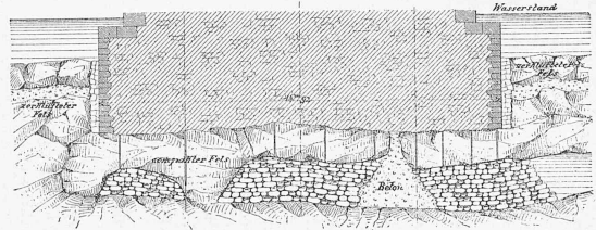
Fig 5. Grundriss des 2 ten Pfeilers
