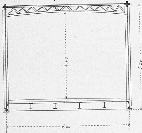
Querschnitt.
