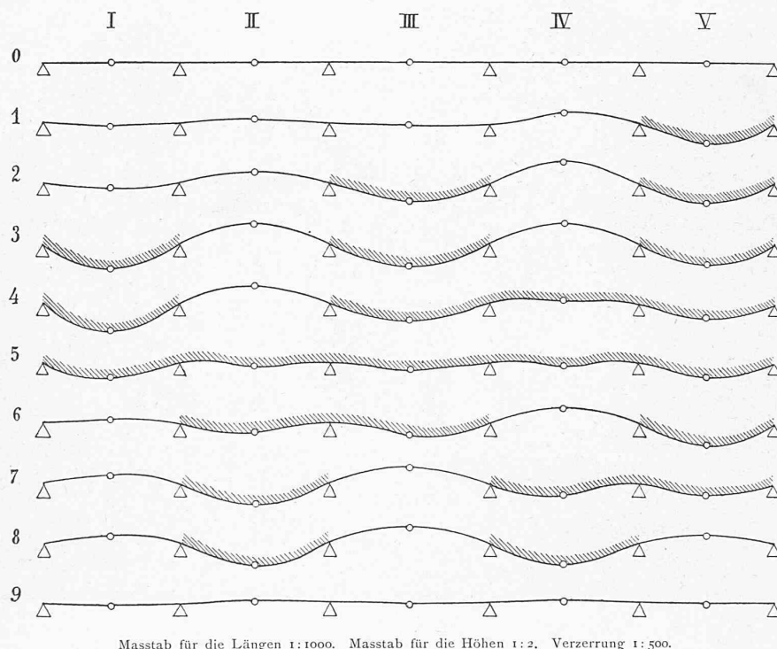
Masstab für die Längen 1:1000. Masstab für die Höhen 1:2. Verzerrung 1:500.
