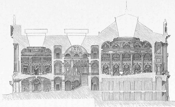
Schnitt. Masstab 1:500.
