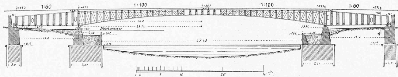
Maßstab 1:500
