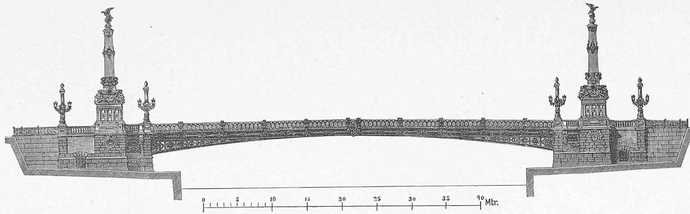
Längenschnitt.
