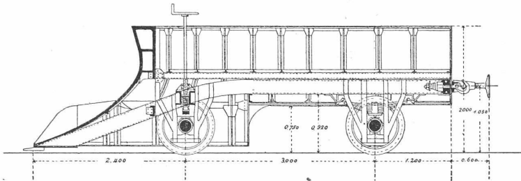
Fig. 1. Längsschnitt ohne Flügel.
