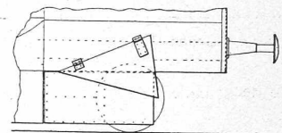
Fig. 10. Flügel, gehört zum eisernen Schneepflug (vide Fig. 5).
