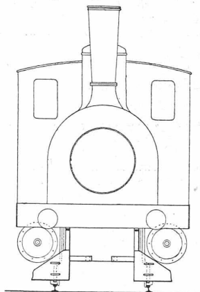
Masstab 1 : 75.
