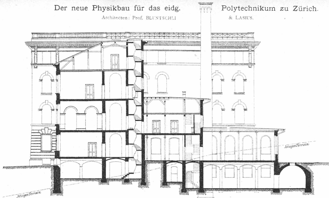
SCHNITT G-H.
