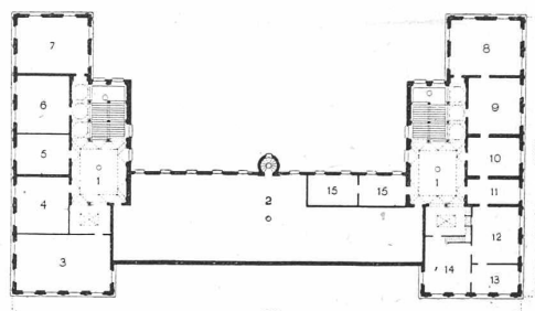
Grundriss vom zweiten Stock.
