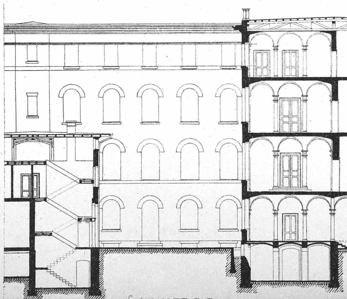
SCHNITT E-F.
