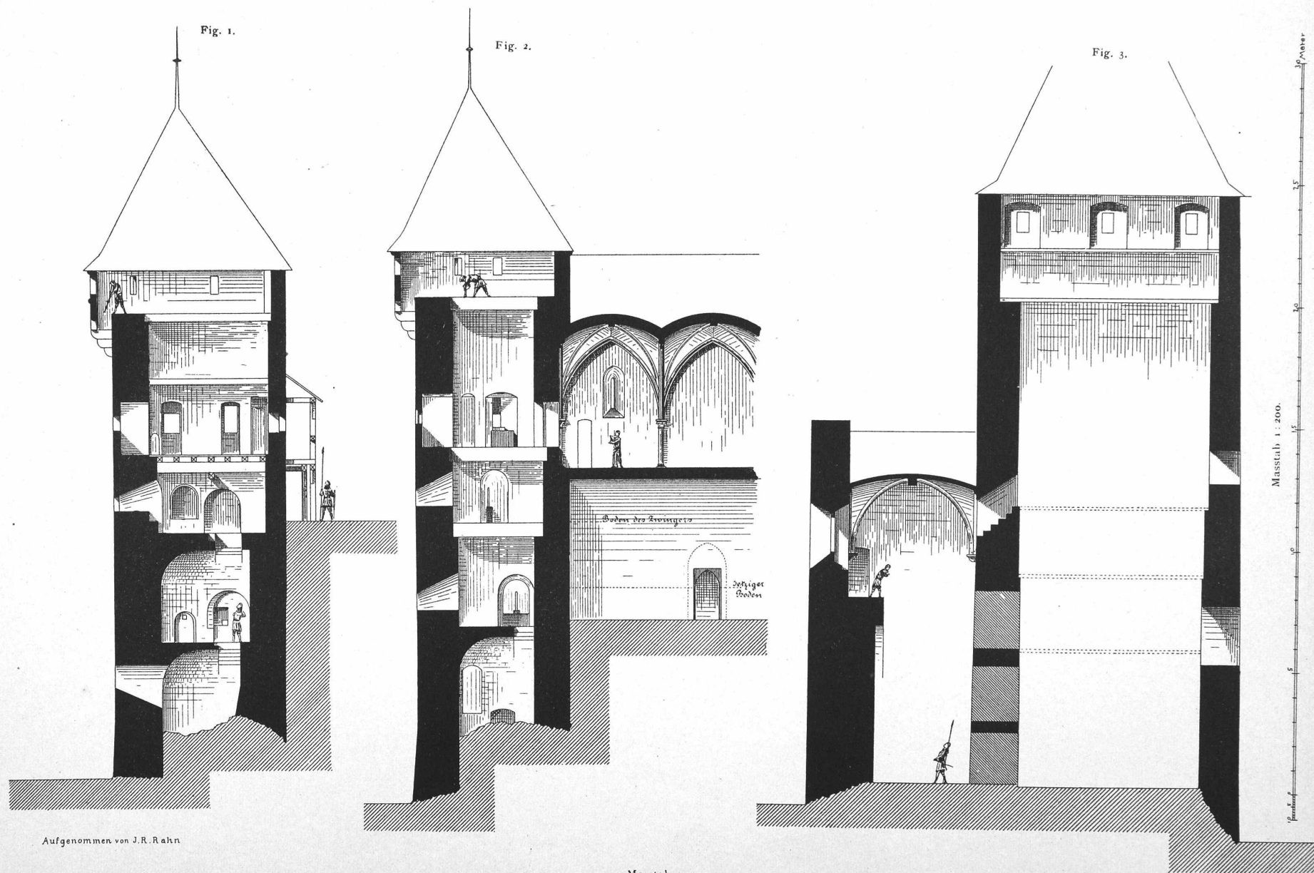
Schnitt durch drei Thürme.
