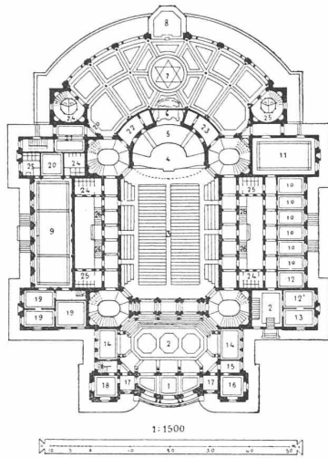
Grundriss vom Erdgeschoss.
