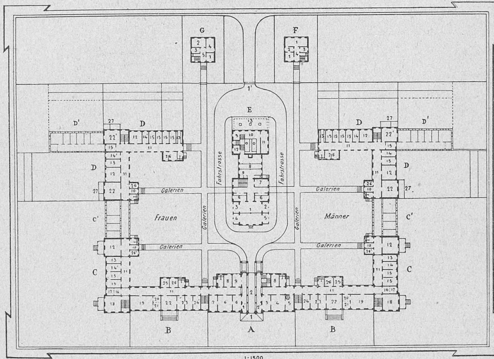
Grundriss vom Erdgeschoss.
