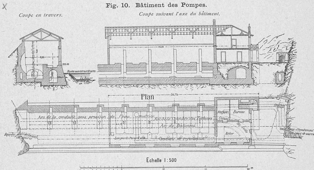
Fig. 10. Bâtiment des Pompes.
