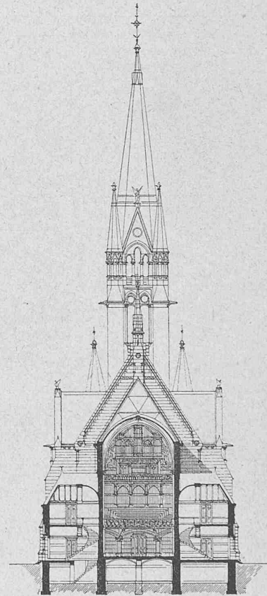
Querschnitt durch den Chor.
