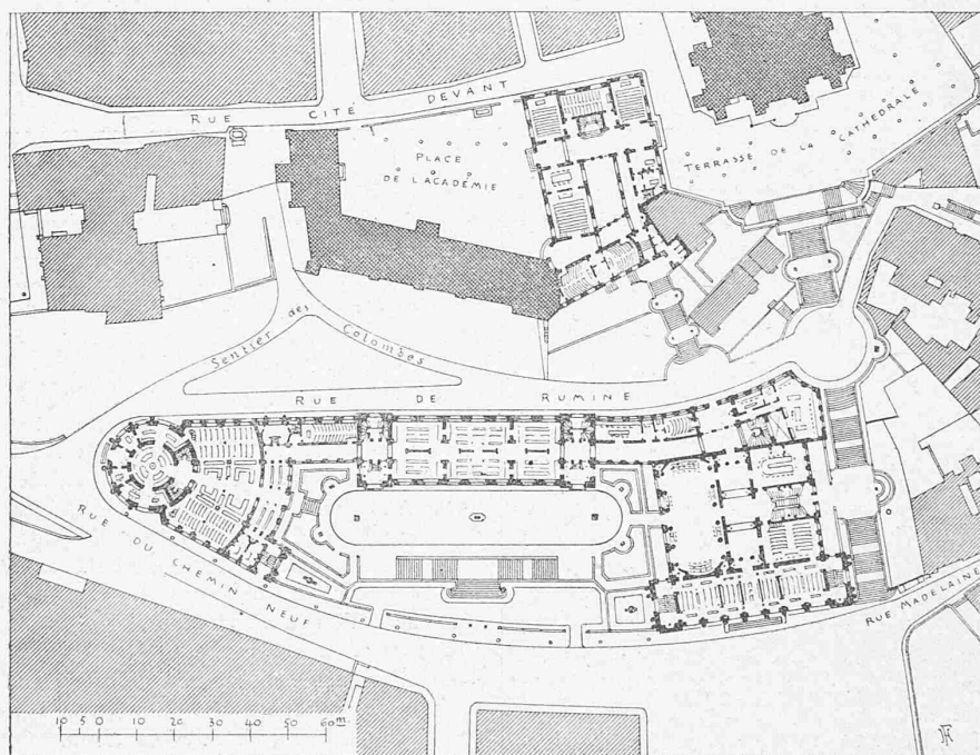
Lageplan und Hauptgrundriss.
