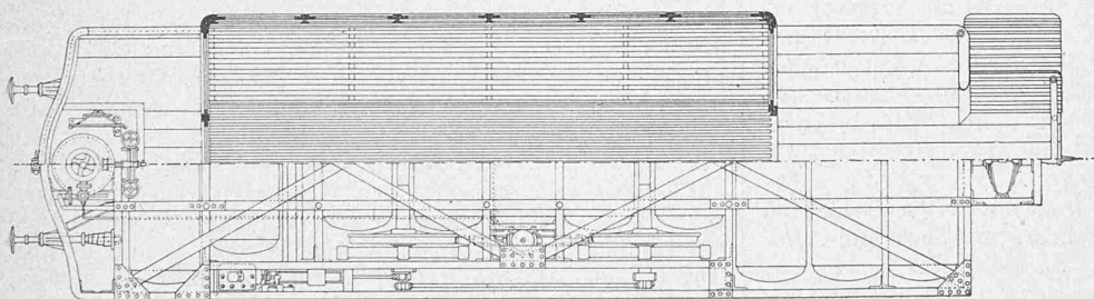
Fig. 5. Grundriss.
