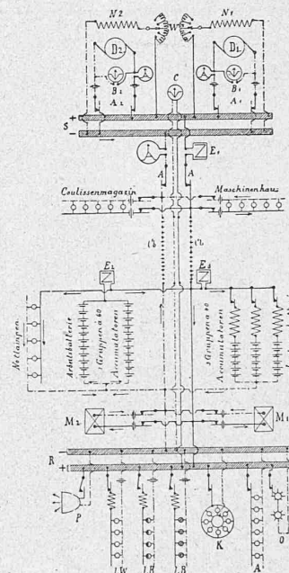
Fig. 2. Schema der electricischen Beleuchtungsanlage im neuen Stadttheater zu Zürich.
