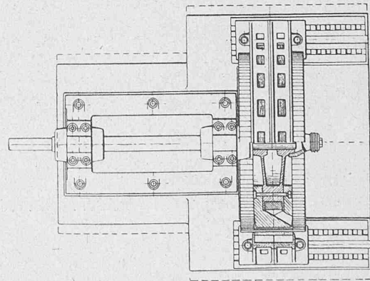
Grundriss. 1 : 50.
