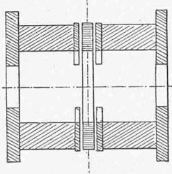
Fig. 5. Flachringmaschine.
