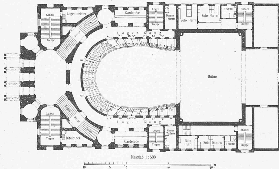
Grundriss vom Zwischengeschoss.
