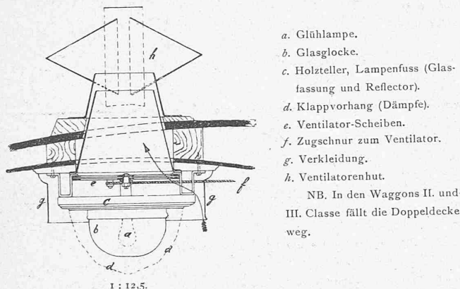
Fig. 2. Ventilator und elektrische Lampe für Wagen der J.-S.-B.
