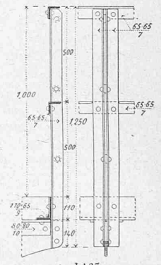
Fig. 8. Geländer.
