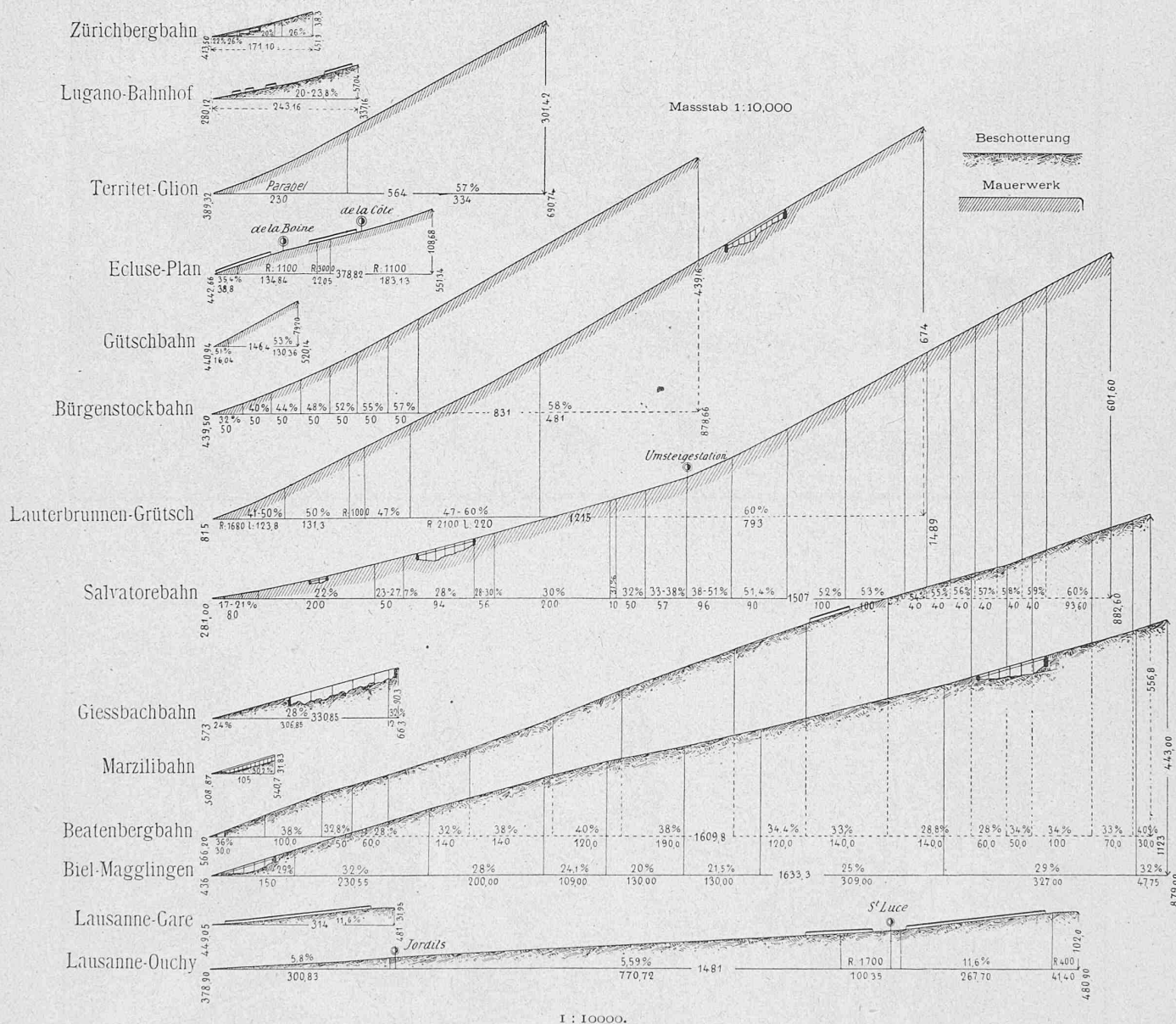
Schweizerische Drahtseilbahnen. Generelle Längenprofile.
