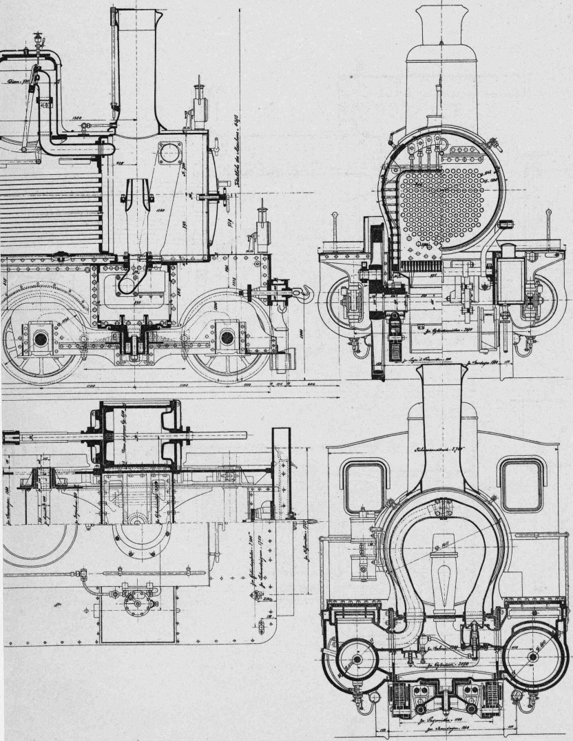
Stab 1:40.
