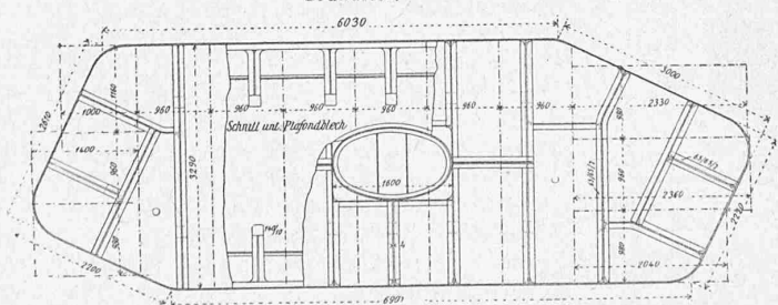
Grundriss.
