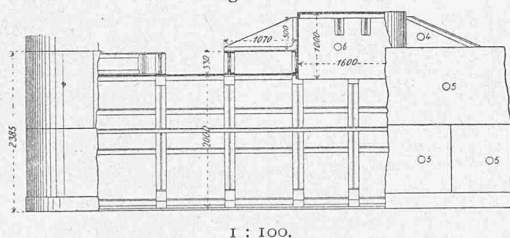
Caisson vom Widerlager II. Rechtes Ufer. Längenschnitt.
