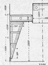
Querschnitt.
