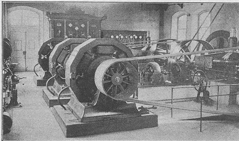
Fig. 2. Maschinenraum.
