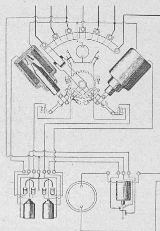
Fig. 4. Automatischer Zellschalter.
