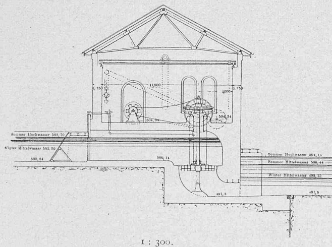
Fig. 3. Maschinenhaus: Querschnitt.
