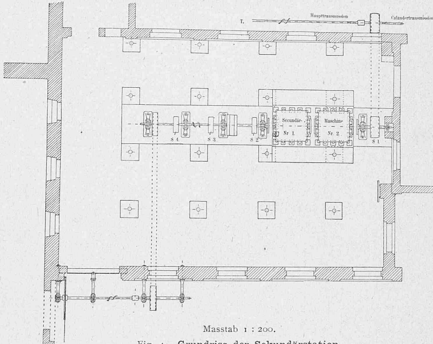
Masstab 1 : 200. Fig. 4. Grundriss der Sekundärstation.
