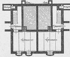
Grundriss III
