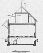
Schnitt IV
