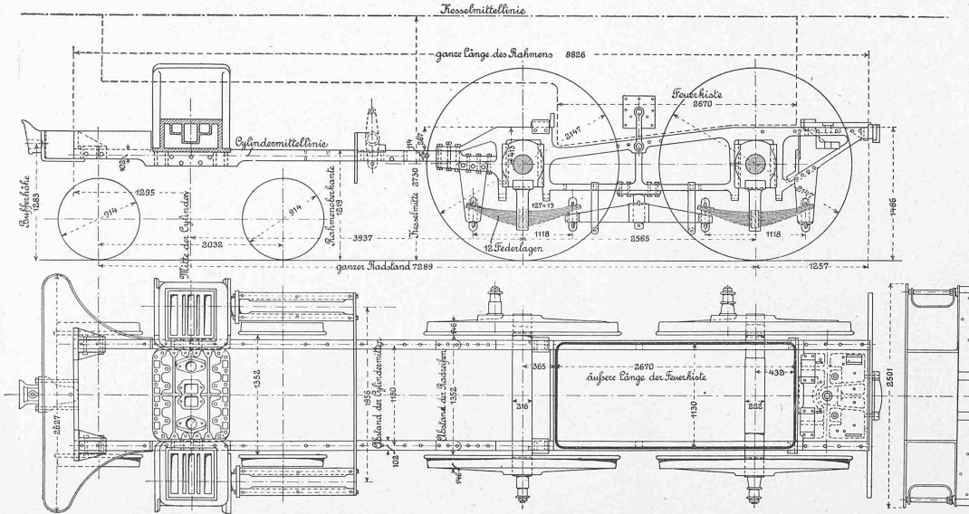
Fig. 5, 6 u. 7. Amerikanische Normal-Konstruktion eines Lokomotivrahmens. — Masstab 1 : 50.
